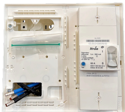
Platine + disjoncteur
