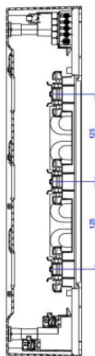
COUPE A-A
