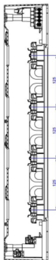
COUPE A-A
